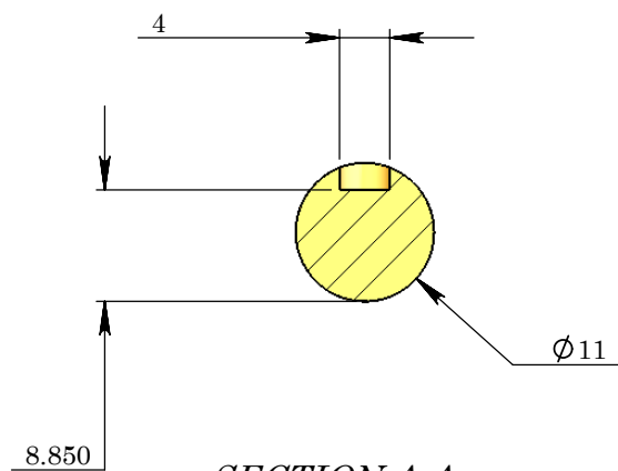
SECTION A-A SCALE 3 : 2
